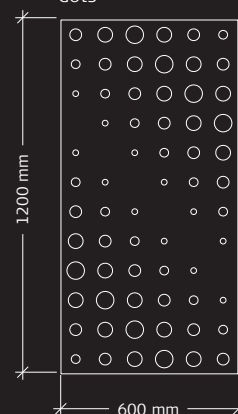
Troldtekt® dots
