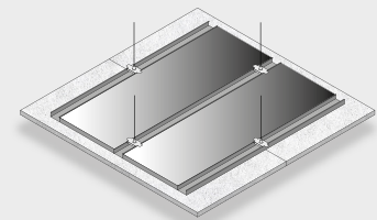
Fig. 3: Acoustic Pads for Troldtekt Elements monteret.
