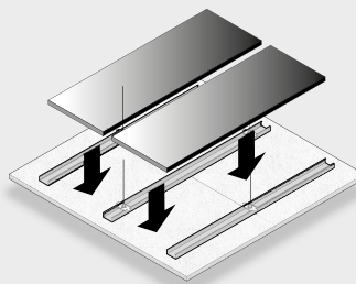
Fig. 2: Acoustic Pads for Troldtekt Elements lægges løst op imellem C60-skinne.
