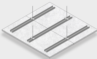
Fig. 1: Troldtekt Elements flådeloftet monteret
