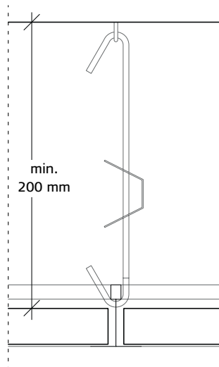
Indbygningshøjde, T35-skiner
