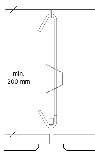
Indbygningshøjde, T35-skinner
